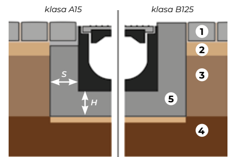
1. Bruk 2. Warstwa wyrównawcza 3. Warstwa nośna 4. Podłoże 5. Beton
